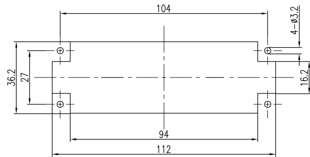
开孔尺寸图
