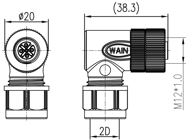
电缆直径:2D5 Cable outlet:2D5
